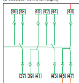
4 переключающих контакта (в базовой комплектации)
