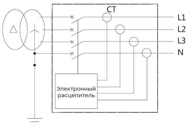
Выключатель исполнением 4P
